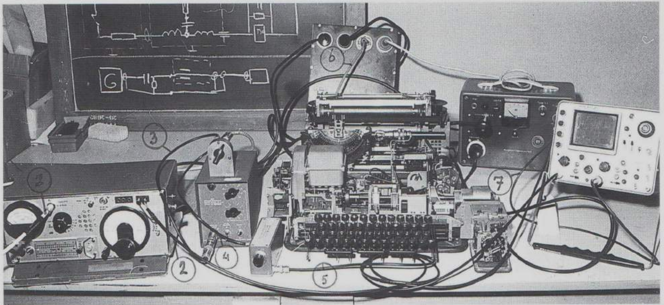
Apparatuur om de straling van telex-apparatuur te meten.
